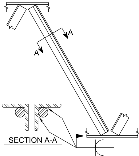
Fig. 15. Rod reinforcing.
